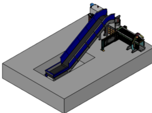
Diseño 3D
